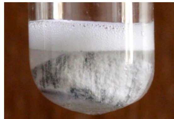
Реакция с мрамором
